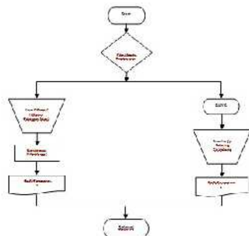
Gambar 2 Flowchart Pembayaran
